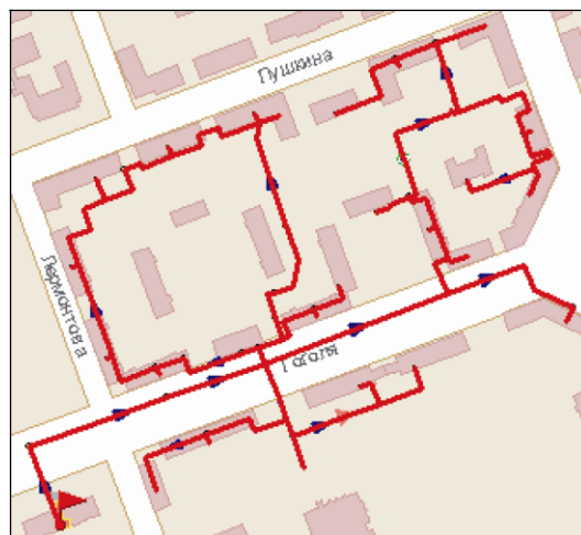
Рисунок 22.2. Нахождение связанных элементов сети
